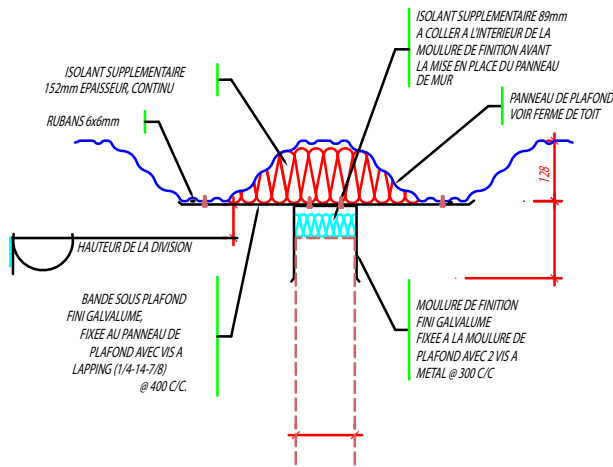
ASSEMBLAGE DE DIVISION INTERIEURE AU PANNEAU DE PLAFOND
