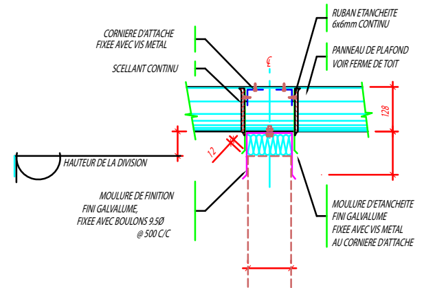
ASSEMBLAGE DE DIVISION INTERIEURE AU PANNEAU DE PLAFOND @ 45°
