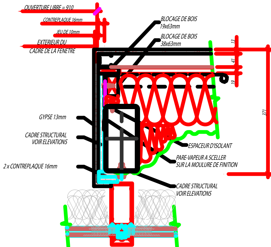
JAMBAGE DOUBLE POUR FENETRE EN ALUMINIUM
